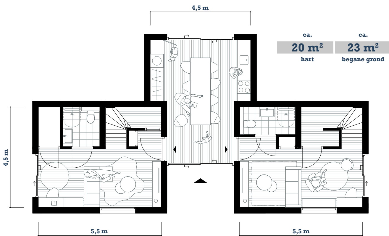
begane grond
